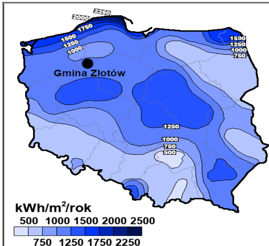
Rysunek 9. Położenie Gminy Złotów na mapie energii wiatru w kWh/m 2 na wysokości 30 m nad poziomem gruntu
